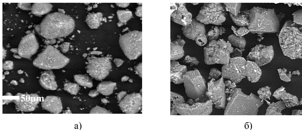
Рис. 1. Структура модифицированных порошков на основе оксида алюминия- оксида циркония: а) - исходный порошок; б) - модифицированный медью
